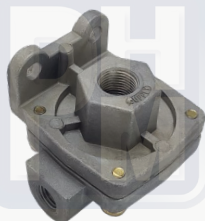
Válvula de liberación rápida
