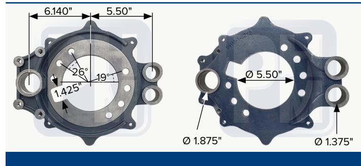
Araña de frenado izquierda, barrenos de Ø 0.656", par de PHM 13212B
