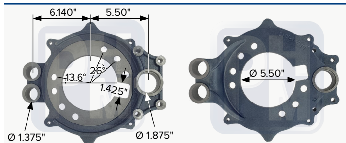
Araña de frenado derecha, barrenos de Ø 0.656", par de PHM 13212G
