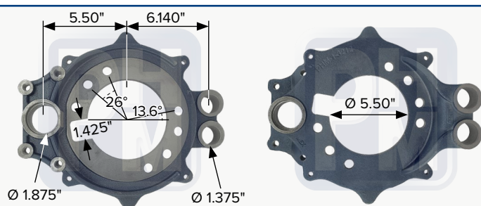
Araña de frenado izquierda, barrenos de Ø 0.656", par de PHM 13212G
