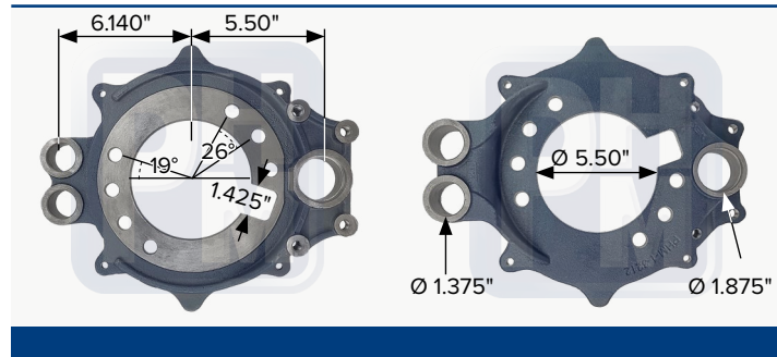
Araña de frenado derecha, barrenos de Ø 0.656", par de PHM 13212A
