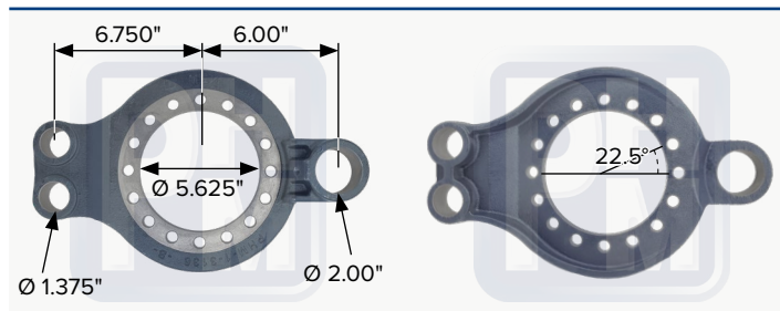
Araña de frenado izquierda o derecha para eje de remolque, de 16 barrenos tipo 1004
