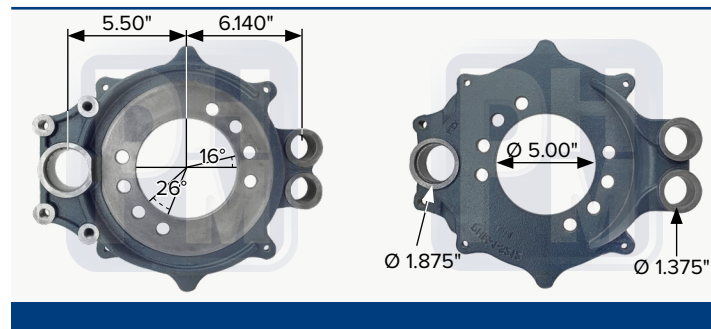
Araña de frenado izquierda, barrenos de Ø 0.656", par de PHM 13212C
