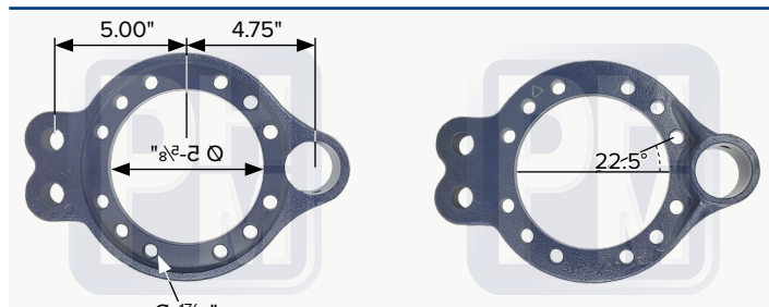
Araña de frenado izquierda o derecha de 12-1/4", para cama baja o low boy
