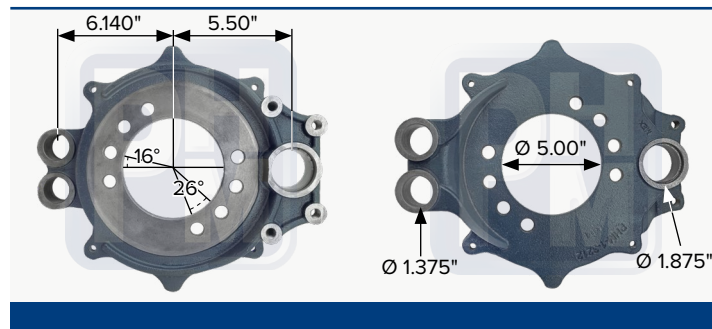
Araña de frenado derecha, barrenos de Ø 0.656", par de PHM 13212K
