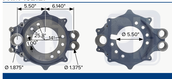
Araña de frenado izquierda, barrenos de Ø 0.656", par de PHM 13212H
