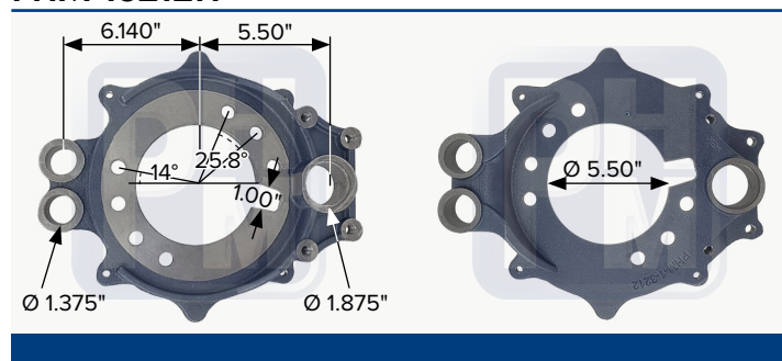
Araña de frenado derecha, barrenos de Ø 0.656", par de PHM 13212I
