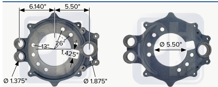
Araña de frenado derecha, barrenos de Ø 0.656", par de PHM 13212L
