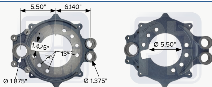
Araña de frenado izquierda, barrenos de Ø 0.656", par de PHM 13212E
