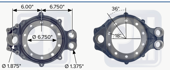
Araña de frenado izquierda o derecha, de 10 barrenos
