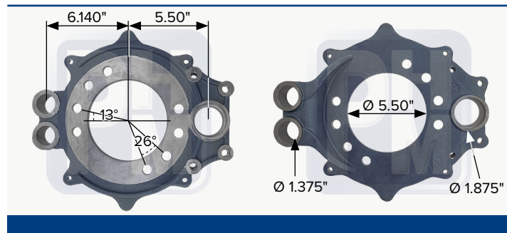
Araña de frenado derecha, barrenos de Ø 0.656", par de PHM 13212J
