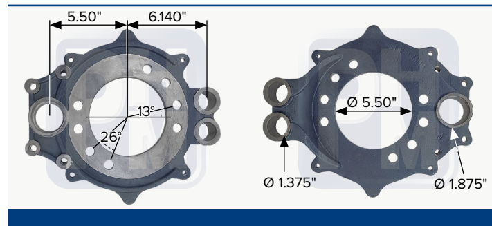
Araña de frenado izquierda, barrenos de Ø 0.656", par de PHM 13212
