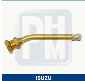
Válvula curva
