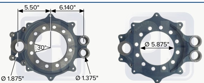
Araña de frenado izquierda o derecha, barrenos de Ø 0.656"
