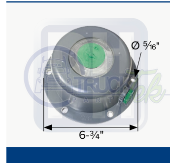
Tapon maza trasera de 6 barrenos
