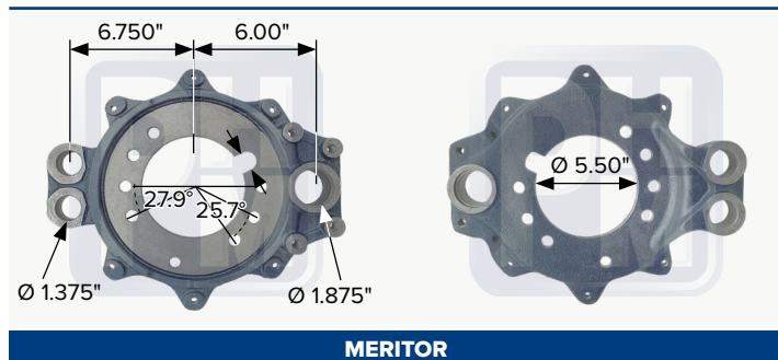
Araña porta zapatas izquierda
