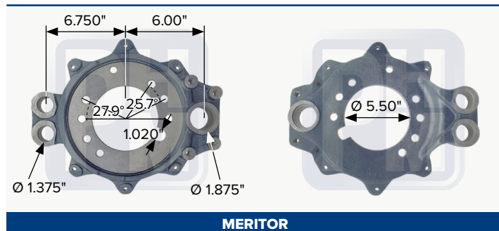
Araña porta zapatas derecha
