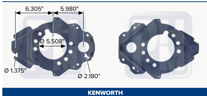
Araña porta zapatas, tipo Bendix
