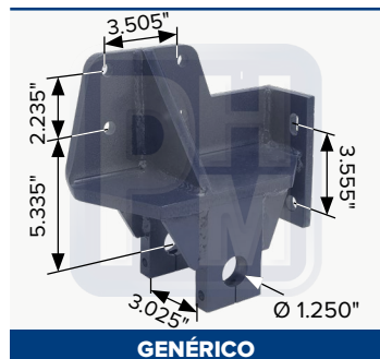
Percha delantera izquierda para suspensión delantera
