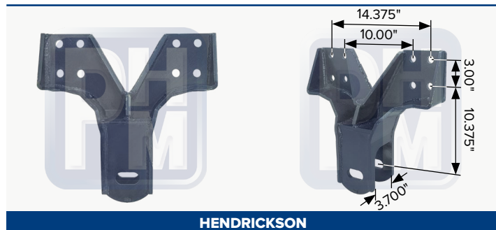
OEM 60784-000, MHS50784 Percha trasera intermedia, para suspensión tipo RTE
