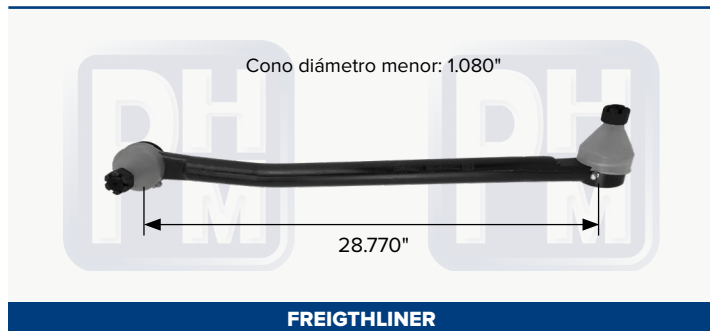
FREIGHTLINER Brazo de dirección con terminales TTES2090 y TTES2091
