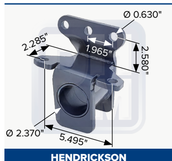
OEM 64176002 Percha derecha tipo AirTek
