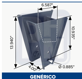
Percha trasera, para remolque, derecha
