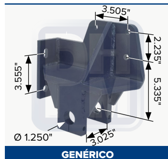
Percha delantera derecha para suspensión delantera
