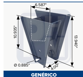
Percha trasera, para remolque, izquierda
