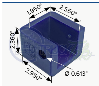
OEM 13-03510 Buje de descanso, para cofre
