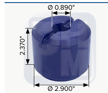
OEM 13-248TBG Tope de rebote para soporte de cofre
