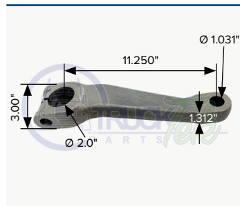
OEM 84242502 Brazo pitman para Kenworth o Peterbilt
