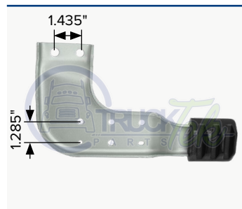
OEM L116131 Guía de cofre izquierda
