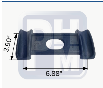
OEM 03-01656, M822 Muelle en U
