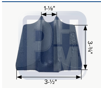
OEM 03-01657, M888 Sobre muelle
