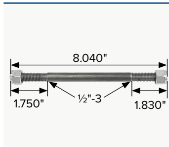
OEM MPB7546, 2701746 Birlo para bolsa de aire
