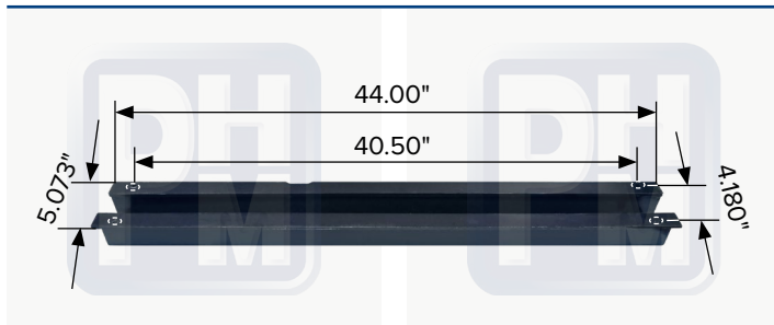
OEM 007-6008, 20582AB Puente para bolsas de aire
